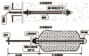
图2 锚索注浆成孔图
